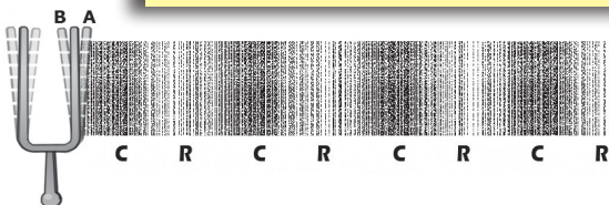
ട്യൂണിങ് ഫോർക്ക് കമ്പനം ചെയ്യുമ്പോൾ വായുവിൽ രൂപപ്പെടുന്ന മർദ്ദവ്യതിയാനങ്ങൾ
